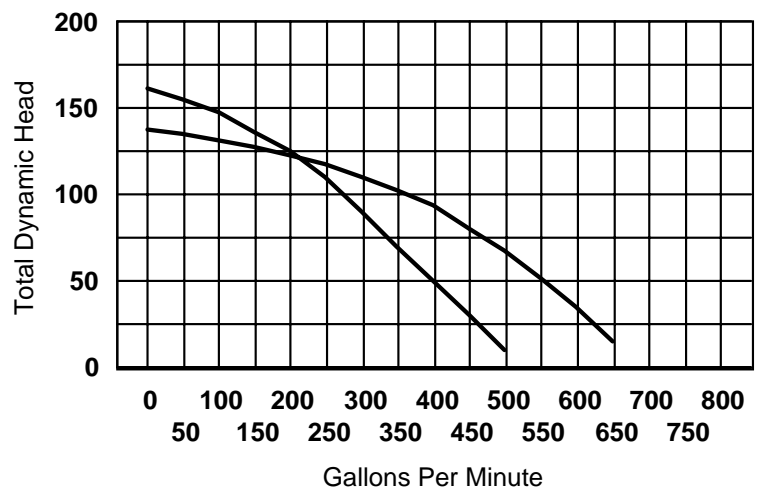
Piranha Model P-1000 HV & HH 10 HP - 230 / 460 V
