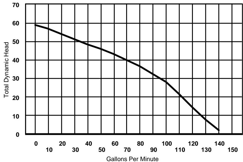
Piranha Model P-150 1.5 HP - 230 / 460 Volt
