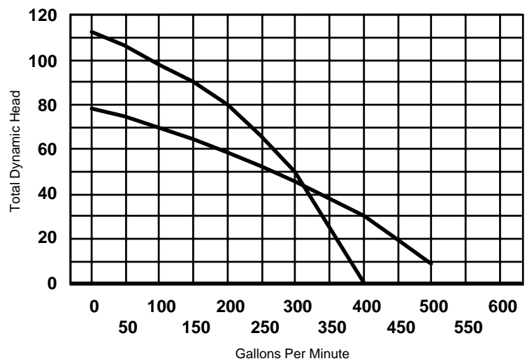
Piranha Model P-650 HV & HH 6.5 HP - 230 / 460 Volt
