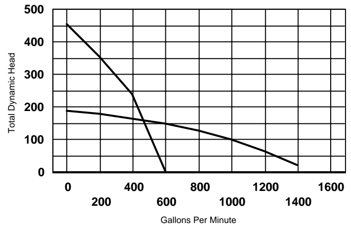
Piranha Model P-4500 HV & HH 45 HP - 460 Volt
